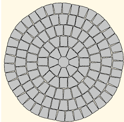
Standardkreis Ø 1540 mm
