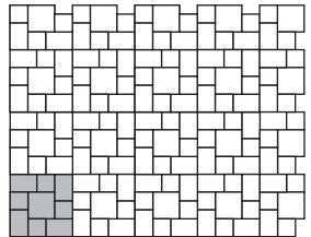
B 8 Steinbedarf pro m 2 120 x 120 x 80 mm 22,7 Stück 180 x 120 x 80 mm 22,7 Stück 180 x 180 x 80 mm 5,7 Stück
