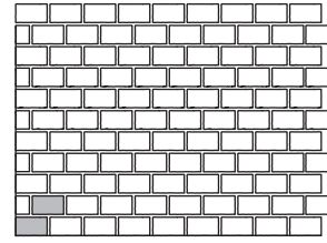
V 1 Steinbedarf pro m 2 208 x 173 x 70 mm 28 Stück
