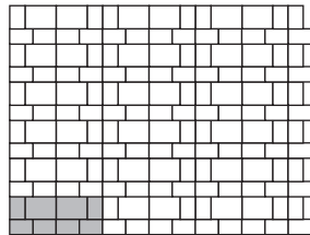
Sa 2 Steinbedarf pro m 2 120 x 180 x 80 mm 27 Stück 240 x 180 x 80 mm 9 Stück
