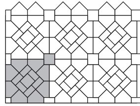
Pa 1 Steinbedarf pro m 2 200 x 200 x 80 mm 5,5 Stück 200 x 100 x 80 mm 9 Stück Diagonalstein 12 Stück
