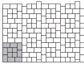
B 2 Steinbedarf pro m 2 120 x 120 x 80 mm 17,4 Stück 180 x 120 x 80 mm 34,7 Stück
