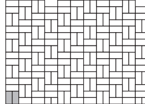
Pa 9 Parkettverband Steinbedarf pro m 2 200 x 100 x 80 mm 50 Stück
