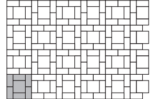
Pa 10 Steinbedarf pro m 2 100 x 200 x 80 mm 37,5 Stück 200 x 200 x 80 mm 6,25 Stück
