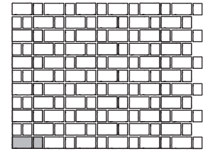
V 5 Steinbedarf pro m 2 208 x 173 x 70 mm 19 Stück 104 x 173 x 70 mm 18 Stück
