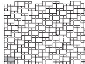
V 6 Steinbedarf pro m 2 208 x 173 x 70 mm 14 Stück 104 x 173 x 70 mm 14 Stück 104 x 86 x 70 mm 28 Stück
