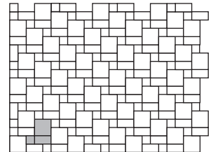
Pa 6 Steinbedarf pro m 2 100 x 100 x 80 mm 14 Stück 100 x 200 x 80 mm 14 Stück 200 x 200 x 80 mm 14 Stück
