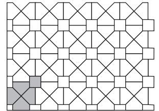
Pa 4 Steinbedarf pro m 2 200 x 200 x 80 mm 3 Stück Diagonalstein 18 Stück
