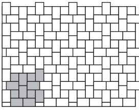
B 1 Steinbedarf pro m 2 120 x 120 x 80 mm 20,0 Stück 180 x 120 x 80 mm 32,5 Stück
