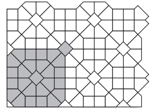
Pa 2 Steinbedarf pro m 2 200 x 200 x 80 mm 8 Stück Diagonalstein 14 Stück
