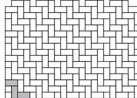
Pa 7 Fischgrätenverband Steinbedarf pro m 2 200 x 100 x 80 mm 50 Stück
