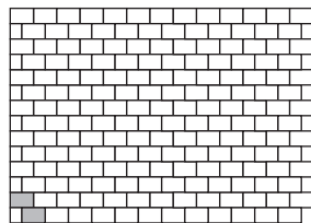
Sa 4 Läuferverband Steinbedarf pro m 2 120 x 180 x 80 mm 48 Stück
