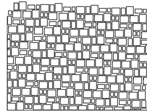
V 2.1 Steinbedarf pro m 2 208 x 173 x 70 mm 20 Stück 104 x 173 x 70 mm 9 Stück 104 x 86 x 70 mm 18 Stück
