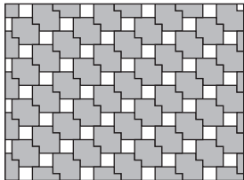
O 5 Steinbedarf pro m 2 200 x 200 x 80 mm 23 Stück 100 x 100 x 80 mm 20 Stück
