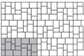
Sa 3 Steinbedarf pro m 2 240 x 180 x 80 mm 13,71 Stück 120 x 180 x 80 mm 18,86 Stück
