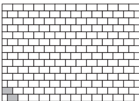
Sa 1 Läuferverband Steinbedarf pro m 2 240 x 180 x 80 mm 24 Stück
