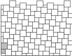
B 5 Steinbedarf pro m 2 120 x 120 x 80 mm 21,4 Stück 180 x 180 x 80 mm 21,4 Stück
