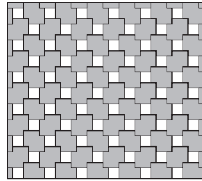
O 4 Steinbedarf pro m 2 200 x 200 x 80 mm 23 Stück 100 x 100 x 80 mm 20 Stück
