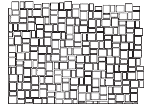
V 2 Steinbedarf pro m 2 208 x 173 x 70 mm 20 Stück 104 x 173 x 70 mm 18 Stück
