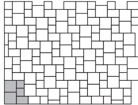
B 6 Steinbedarf pro m 2 120 x 120 x 80 mm 17,4 Stück 180 x 120 x 80 mm 8,7 Stück 180 x 180 x 80 mm 17,4 Stück
