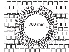
V 13 Steinbedarf für Einfassung Schachtdeckel (3 Ringe) 104 x 173 x 70 mm 36 Stück 104 x 86 x 70 mm 59 Stück Steinbedarf pro m 2 für Flächenverlegung 208 x 173 x 70 mm 28 Stück
