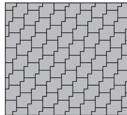
O 6 Steinbedarf pro m 2 200 x 200 x 80 mm 28,5 Stück
