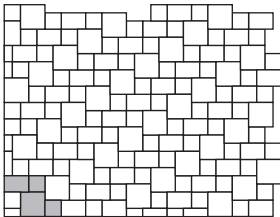
B 7 Steinbedarf pro m 2 120 x 120 x 80 mm 24,2 Stück 180 x 120 x 80 mm 12,1 Stück 180 x 180 x 80 mm 12,1 Stück
