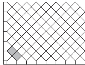
Pa 3 Steinbedarf pro m 2 200 x 200 x 80 mm 25 Stück Steinbedarf pro lfm. Diagonalstein 3,5 Stück
