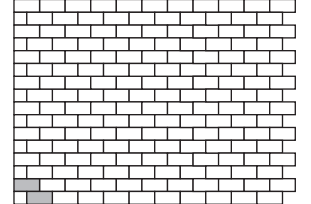
Pa 8 Läuferverband Steinbedarf pro m 2 200 x 100 x 80 mm 50 Stück
