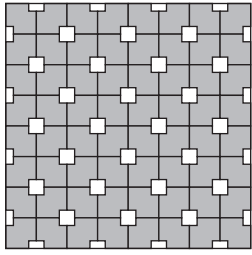
O 1 Steinbedarf pro m 2 200 x 200 x 80 mm 25 Stück 100 x 100 x 80 mm 12,5 Stück
